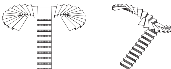
teilgewendelte Treppen symmetrisch mit einem geraden Antrittsarm und zwei gewundenen Austrittsarmen
